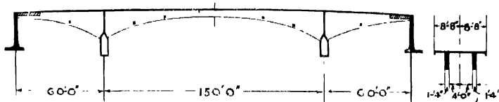
Fig. 346. Longitudinal Section.
